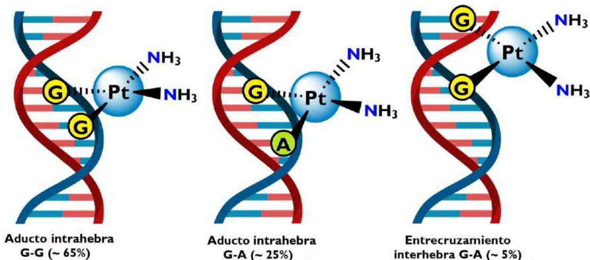
Figura 2. Mecanismo de acción del cisplatino coordinado con las bases nitrogenadas del ADN. Figure 2. Mechanism of action of cisplatin coordinated with the nitrogenous bases of DNA.
