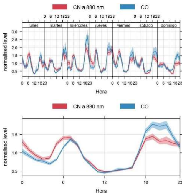
Figura 4. Tendencia de CN y CO en lapsos de una semana y de 24 horas. El sombreado representa 95% de intervalo de confianza determinado a través del método bootstrap resampling, integrado en la función Time Variation de OpenAir.
