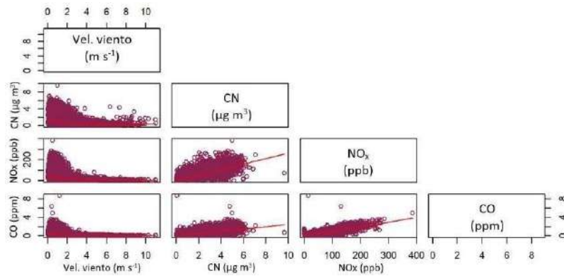
Figura 5. Gráfica de dispersión entre CN, CO, NO x y velocidad de viento, cada una corresponde a la intersección entre las variables indicadas.
