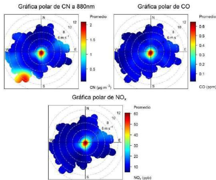
Figura 6. Gráficas polares de CN, CO y NO x , comparadas con dirección y velocidad de viento.
