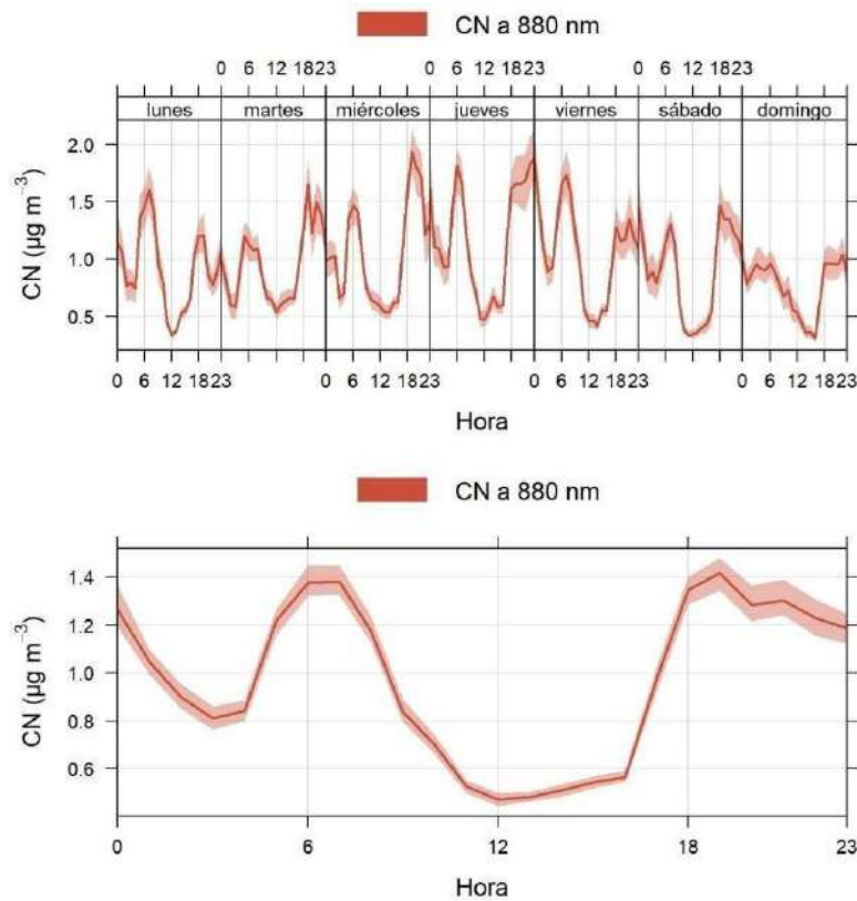
Figura 2. Tendencia de CN en lapsos de una semana y de 24 horas. El sombreado representa 95% de intervalo de confianza, determinado a través del método bootstrap resampling, integrado en la función Time Variation de OpenAir.
