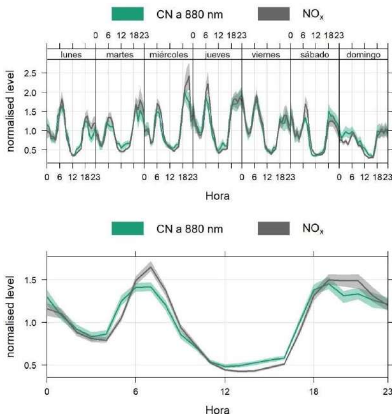
Figura 3. Tendencia de CN y \text{NO}_x en lapsos de una semana y de 24 horas. El sombreado representa 95% de intervalo de confianza determinado a través del método bootstrap resampling, integrado en la función Time Variation de OpenAir.
