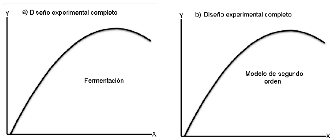
Figura 1. Modelo de fermentación y modelo de segundo orden.
