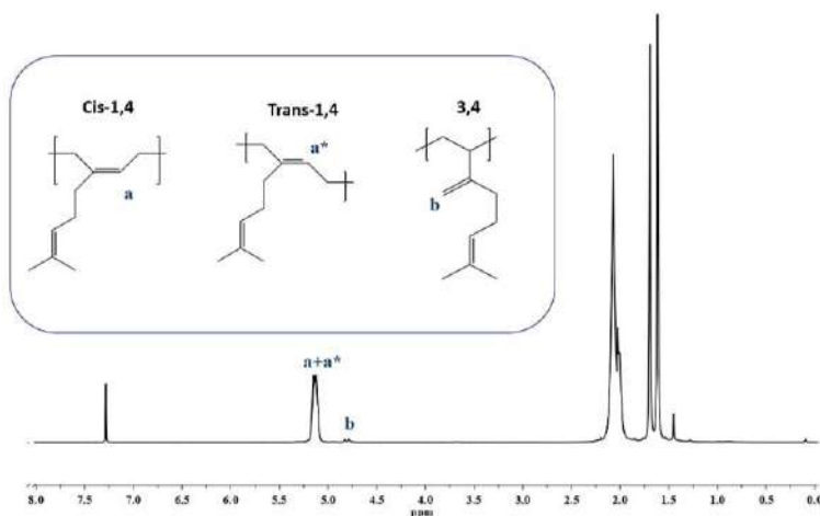
Figura 7. Espectro de ^1\text{H} -NMR de un polimirceno Figure 7. ^1\text{H} -NMR spectrum of a polymyrce
