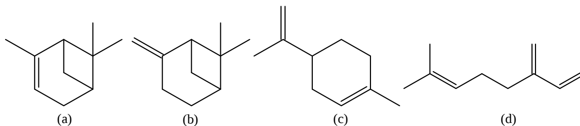
Figura 1. Estructuras químicas de (a) \alpha -pineno, (b) \beta -pineno, (c) limoneno y (d) mircenno (Espinosa Andrews et al. , 2016)
