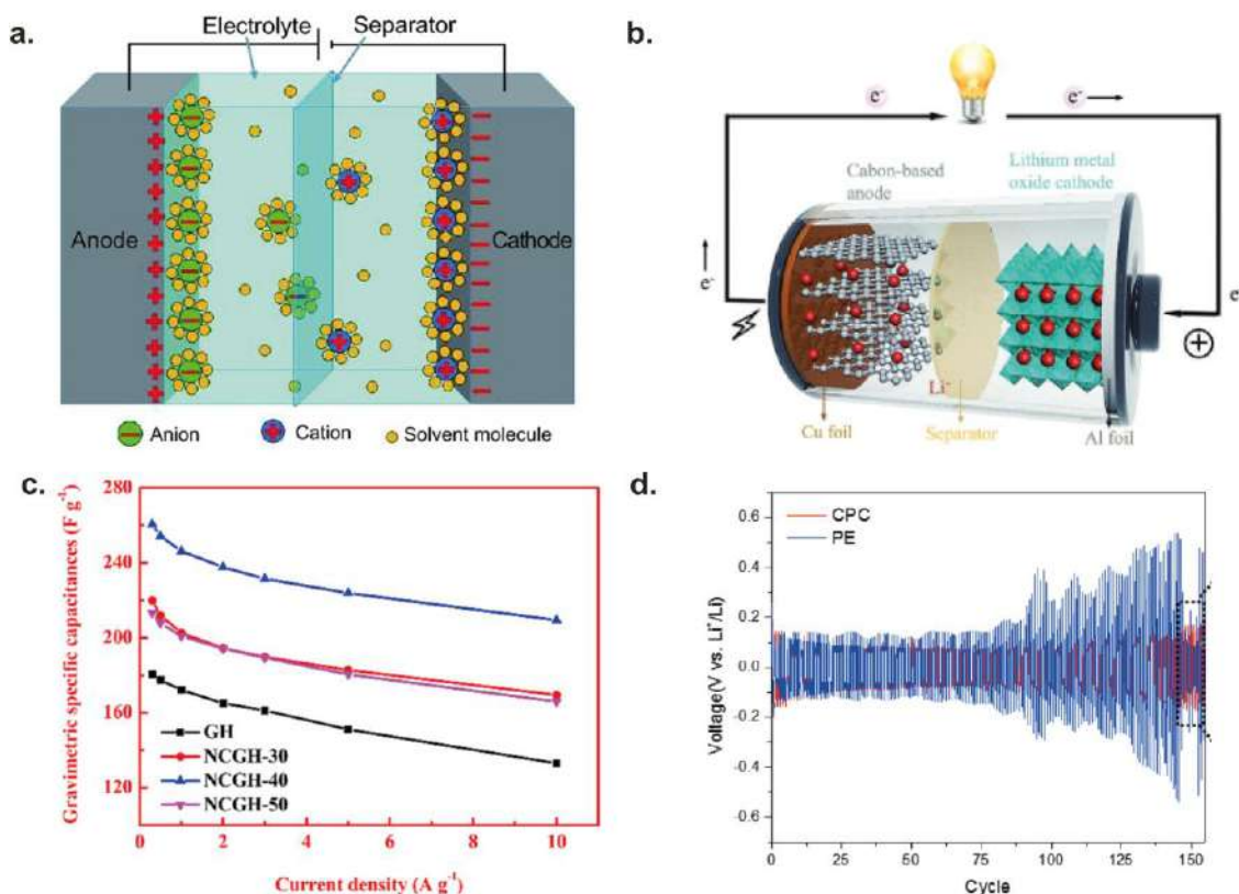
Figure 4. a. Energy storage mechanism in conventional supercapacitors (Copyright 2022, Wiley) (Ali et al. , 2022); b. Energy storage mechanism in conventional lithium-ion batteries (Copyright 2020, Wiley) (Zhang et al. , 2020); c. Capacitance comparison of reduced graphene oxide (GH) and nanocellulose/reduced graphene oxide composite hydrogels (NCGHs) with various loading contents of cellulose nanofibrils (Copyright 2022, American Chemical Society) (Zhang et al. , 2022); d. Performance comparison of lithium-ion batteries consisting of commercial separator (PE) and CNF polyethylene composite (CPC) (Copyright 2018, Wiley) (Pan et al. , 2018). Figura 4. a. Mecanismo del almacenamiento de energía en supercondensadores convencionales (Copyright 2022, Wiley) (Ali et al. , 2022); b. Mecanismo del almacenamiento de energía en baterías de iones de litio convencionales (Copyright 2020, Wiley) (Zhang et al. , 2020); c. Comparación de la capacitancia de hidrogeles compuestos de óxido de grafeno reducido (GH) y nanocelulosa/óxido de grafeno reducido (NCGH) con diversos contenidos de carga de nanofibrillas de celulosa (Copyright 2022, American Chemical Society) (Zhang et al. , 2022); d. Comparación del rendimiento de baterías de iones de litio formadas por un separador comercial (PE) y un compuesto de polietileno CNF (CPC) (Copyright 2018, Wiley) (Pan et al. , 2018).
