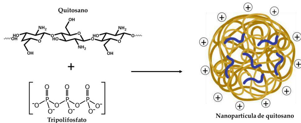
Figura 4. Esquema general del proceso de fabricación de nanopartículas por entrecruzamiento iónico.
