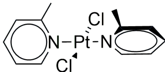
Figura 11. Complejo cuadrado plano de platino con quiralidad axial.
