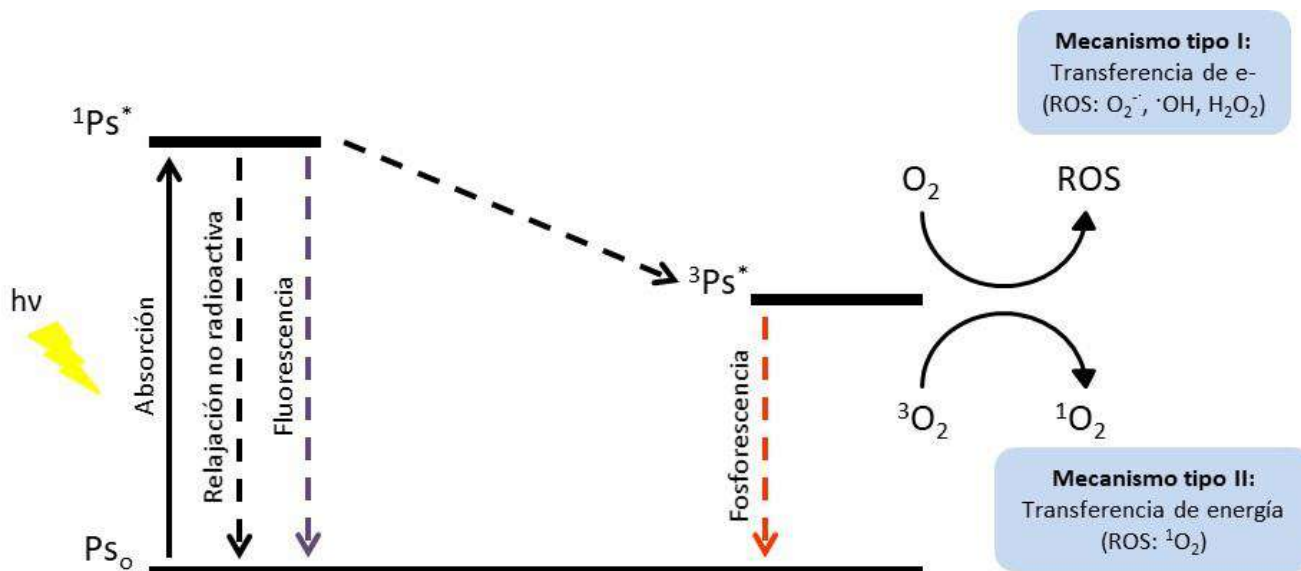
Figura 2. Mecanismos de acción de tipo I y II de la terapia fotodinámica. \text{PS}_0 es el fotosensibilizador en su estado fundamental, ^1\text{PS}^* el fotosensibilizador en su estado excitado singulete, y ^3\text{PS}^* el fotosensibilizador en su estado excitado triplete (O'Connor et al. , 2009).
