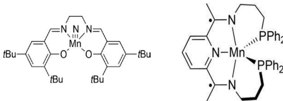
Figura 5. Ejemplos de compuestos de manganeso con ligantes polidentados usados en reducción catalítica.
