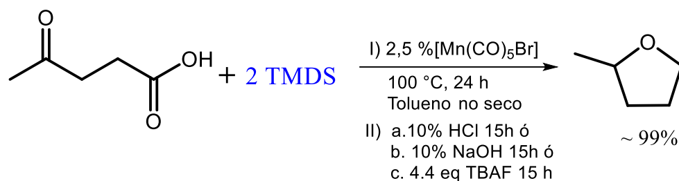
Figura 6. Ejemplo de reducción y ciclación con manganeso. Figure 6. Example of reduction and cyclization with manganese.
