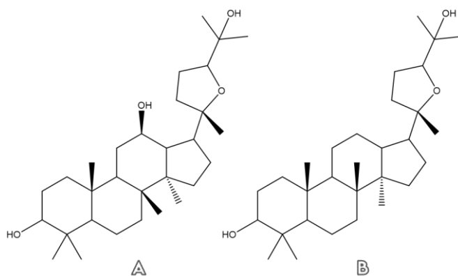
Figura 8. Moléculas de Pyxinol (A) y el Ocotillol (B) presentes en los tallos del ocotillo
