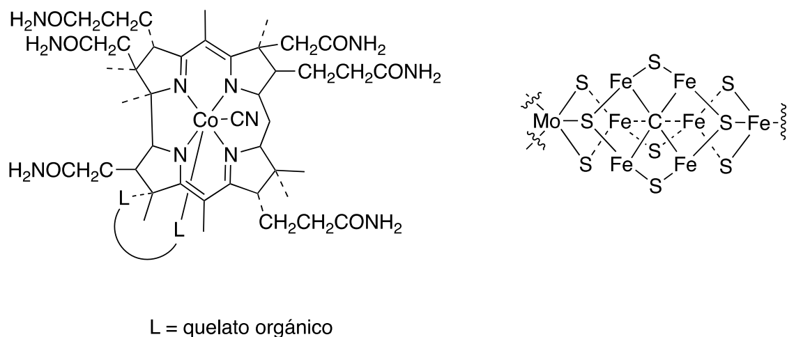
Figura 2. Vitamina B-12 y el cofactor más estudiado de la nitrogenasa (cofactor MoFe).
