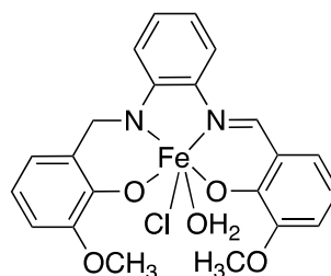
Figura 4. a) Cisplatino y derivados usados para el tratamiento de diferentes tipos de cáncer. b) metalofármacos actualmente en pruebas en fase clínica, auranofin usada también para el tratamiento de la artritis, c) metalofármacos de Fe que son candidatos para usar como agentes contra el cáncer: izquierda (organometálico): utilizado en terapia fotodinámica, derecha (de coordinación): induce apoptosis bloqueando la fase de síntesis en el ciclo celular de células cancerosas.
